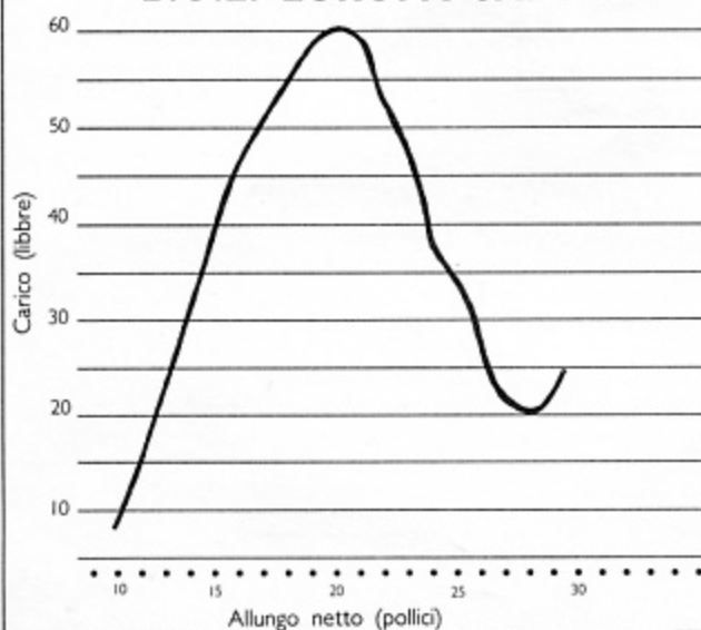
Diagramma di trazione B.O.E. EUROPA SARACEN
