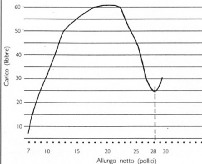
Diagramma di trazione CARBON EXTREME
