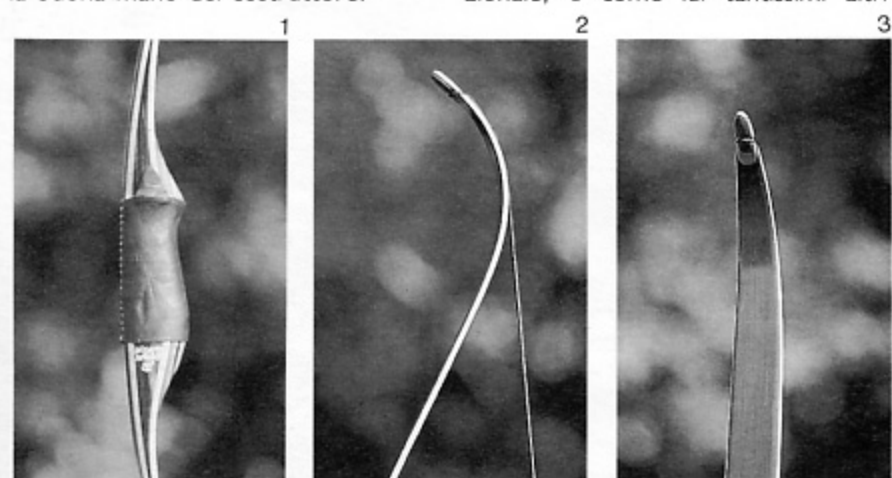
1 l'impugnatura del flatbow ricurvo «legacy». 2 e 3 l'estremità dei suoi flettenti. 4 il fronte del «legacy».
