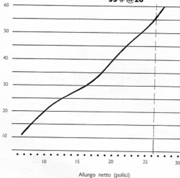
Diagramma di trazione LARRY NIRK «LEGACY» 55# @28"
