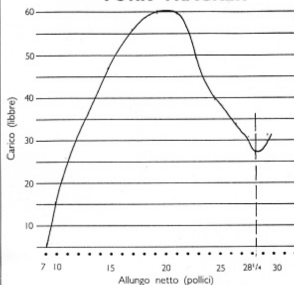
Diagramma di trazione YORK TRACKER
